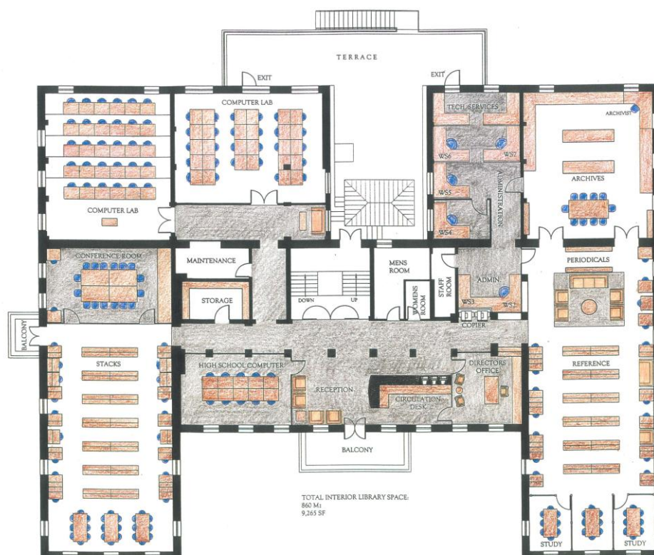
Σχέδιο κάτοψης
